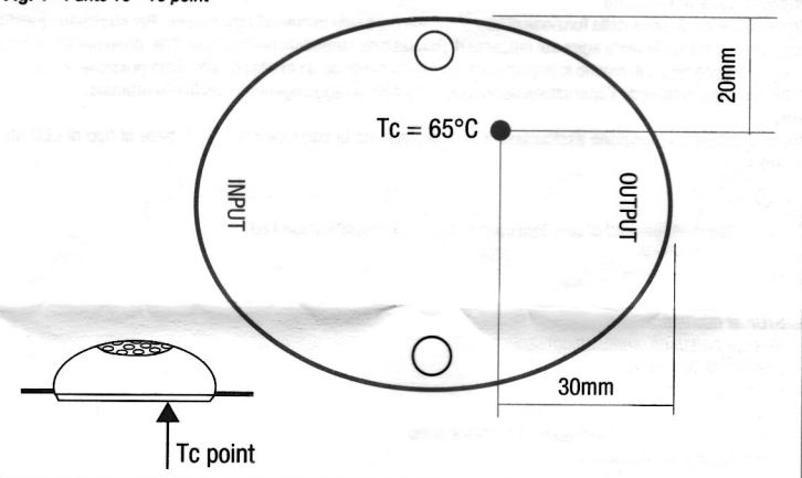
Fig. 4 - Punto Tc - Tc point
