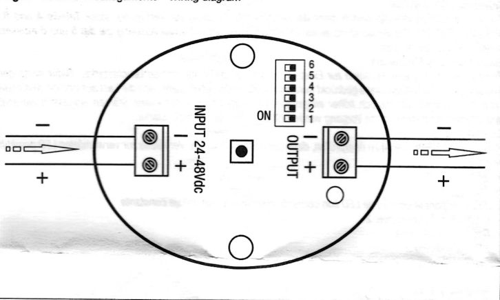
Fig. 3 - Schema di collegamento - Wiring diagram
