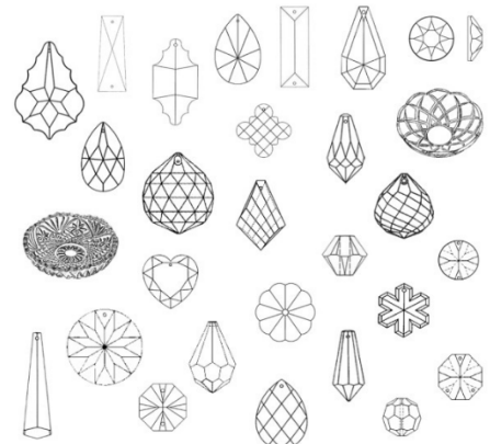
BEGRIFFSERKLÄRUNG – KRISTALLFORMEN
